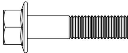
M10-1.25 x 45mm Lg. FHCS
